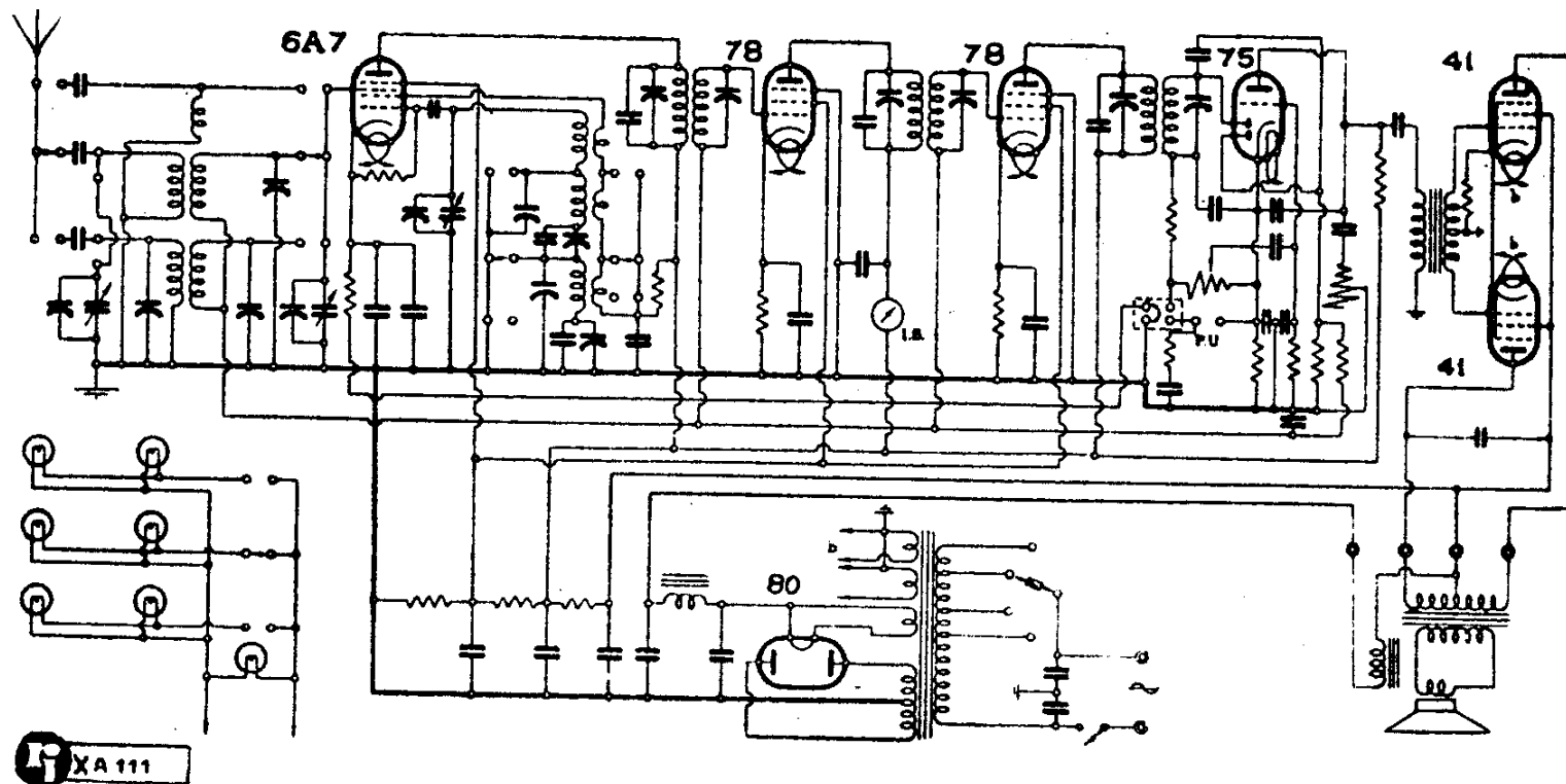
ALLOCCHIO, BACCHINI & C. - MODD. « 75 », « 751 »
